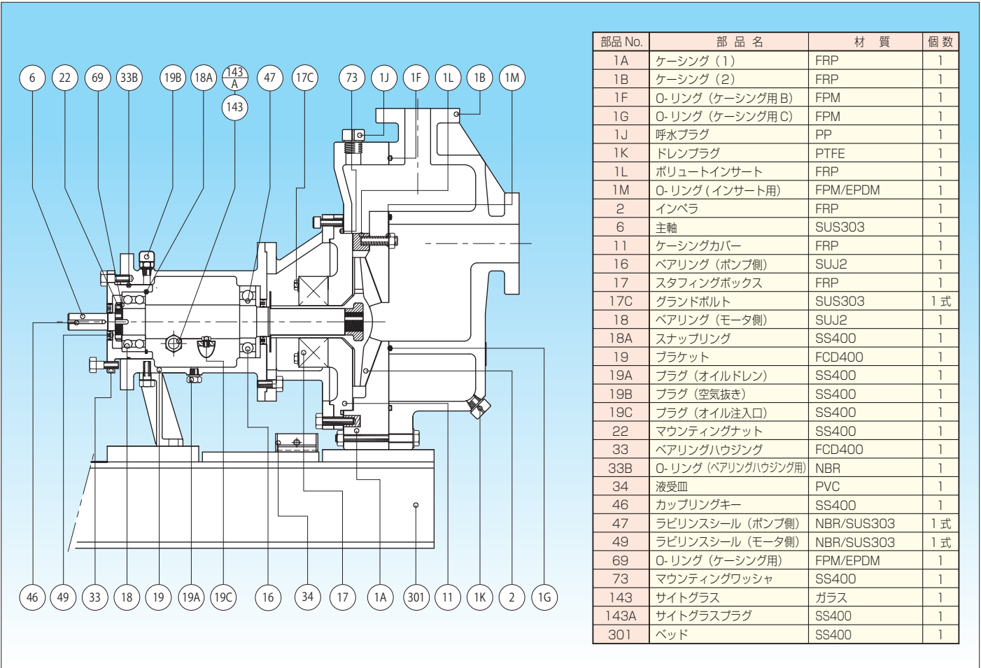
断面構造図
