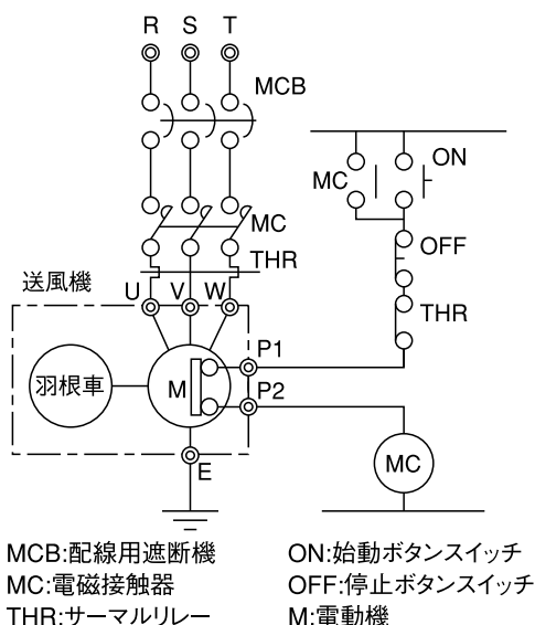
結線の例
