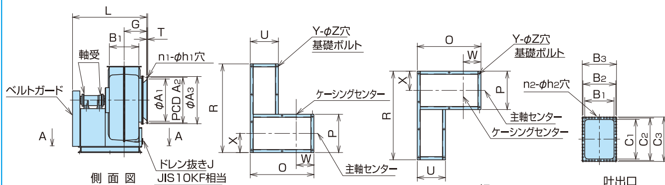
A-A視 RH1,RR1,LH1,LL1,LR1形 基礎図
