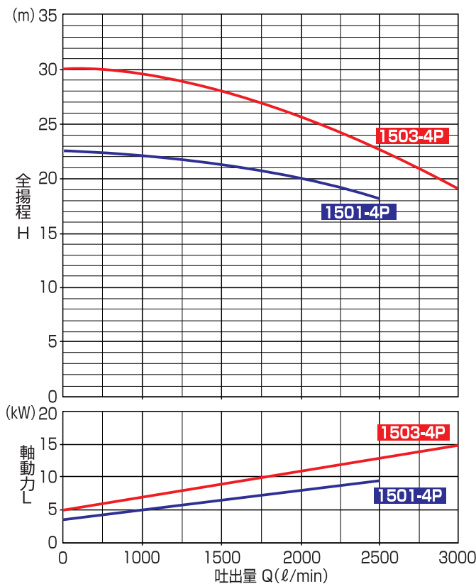
50Hz 性能曲線・要目表
