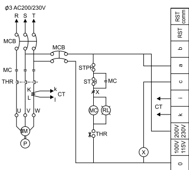
図2 警報回路例
