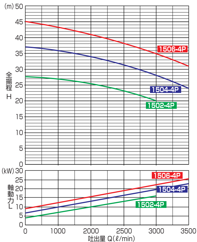
60Hz 性能曲線・要目表
