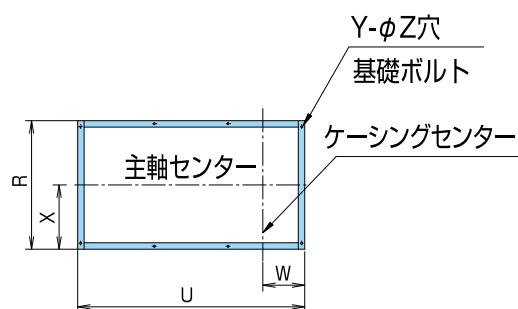
A-A矢視
