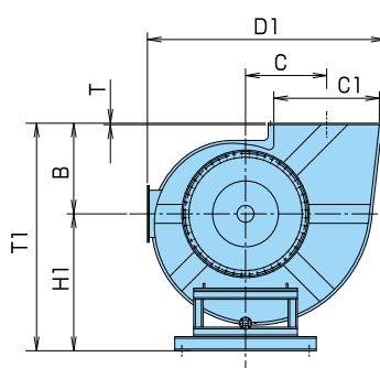
RH形
