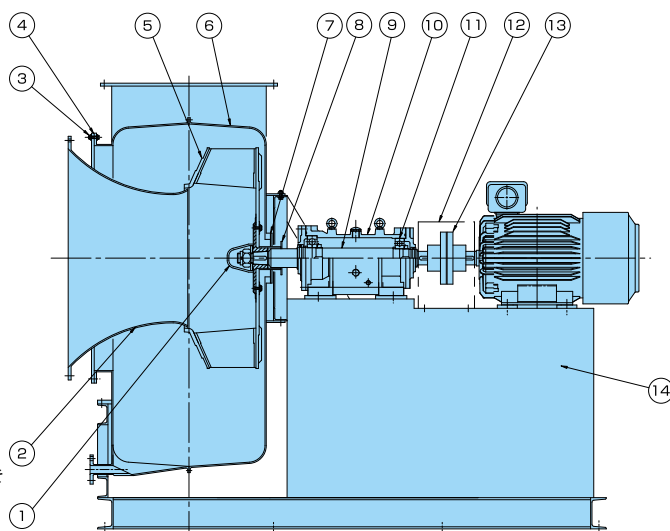
■材質表
