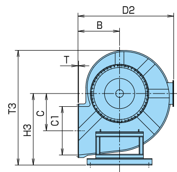
LR形
