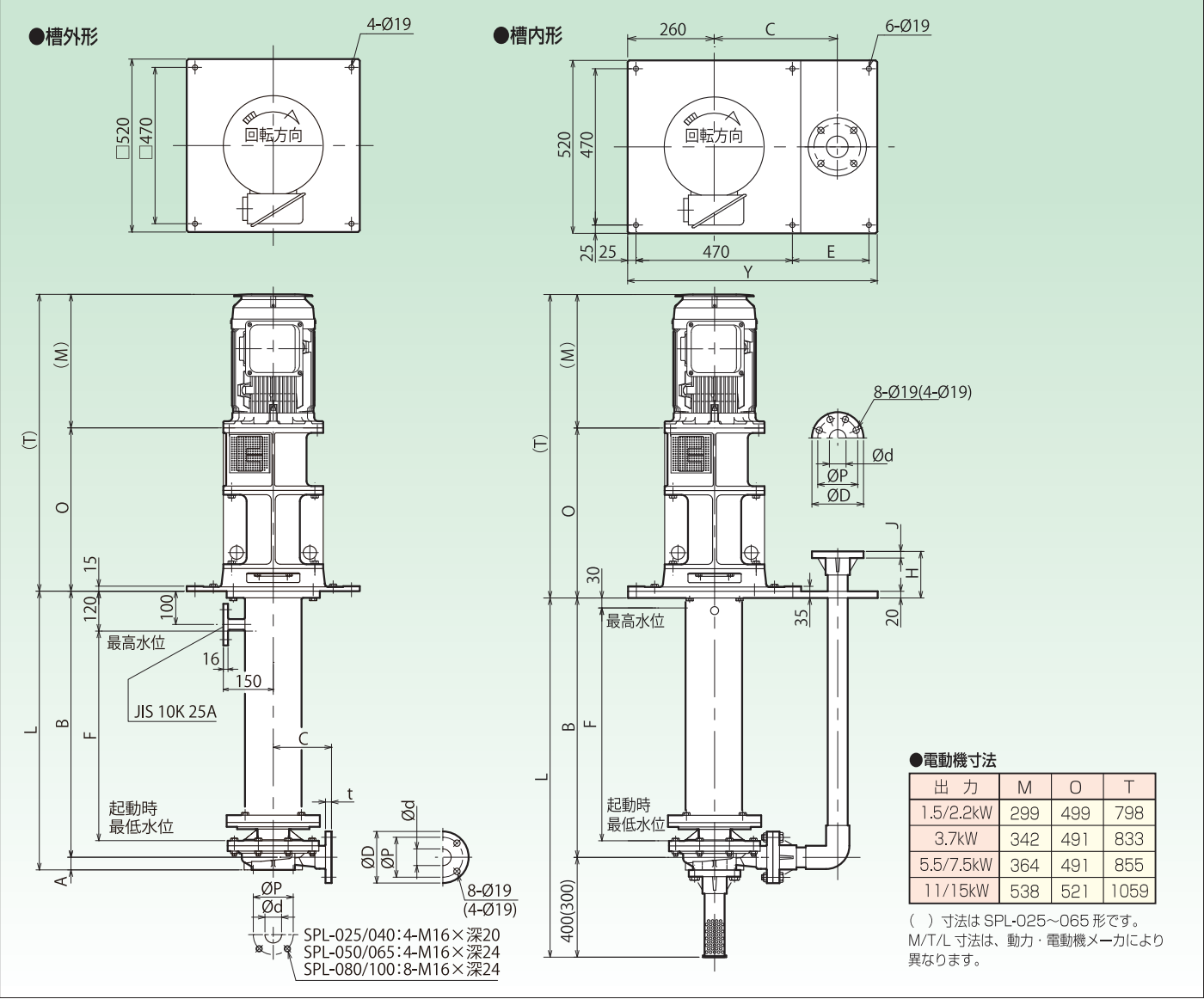
■寸法図
