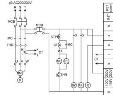
図2 警報回路例
