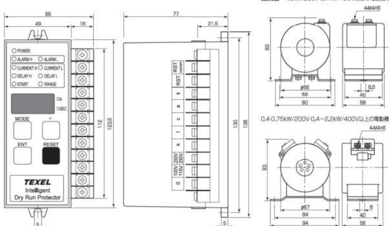
図4 外形寸法図
