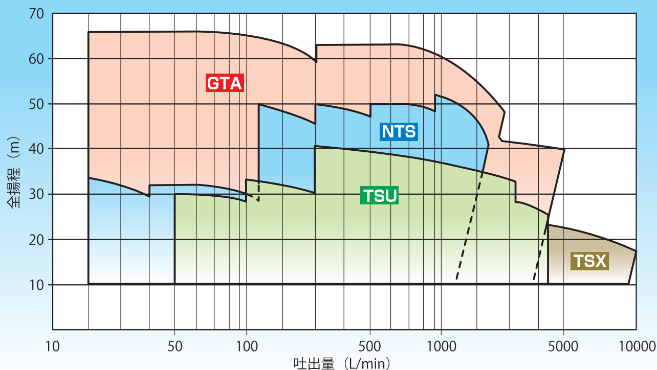
横形ポンプ 60Hz 容量図 〈GTA/TSX/NTS/TSU〉
