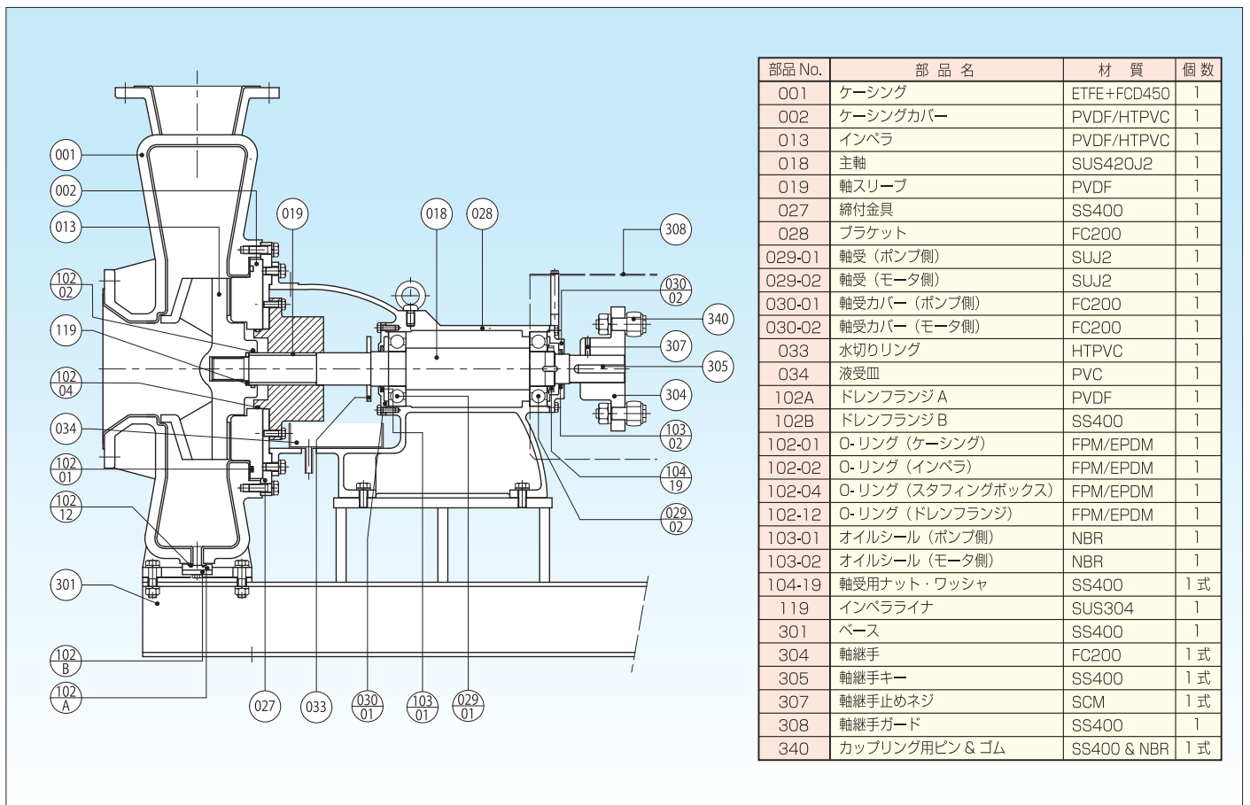
断面構造図
