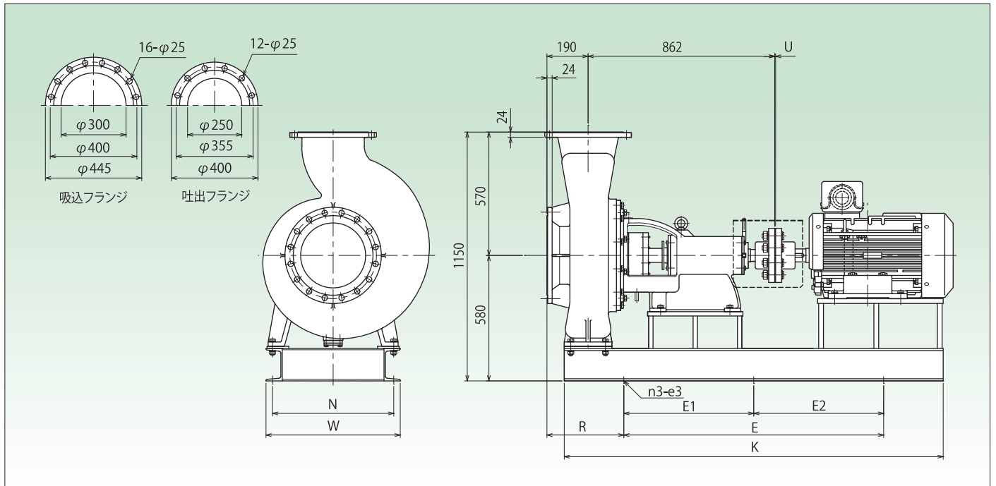
外形寸法図表
