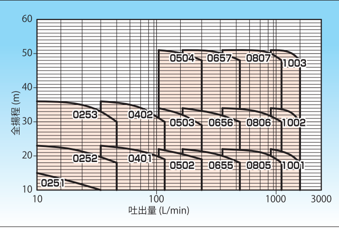
〈2P〉 50Hz 容量図・要目表
