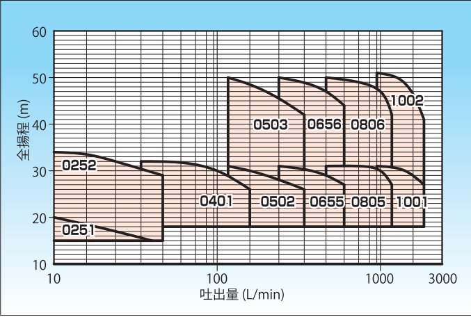
〈2P〉 60Hz 容量図・要目表
