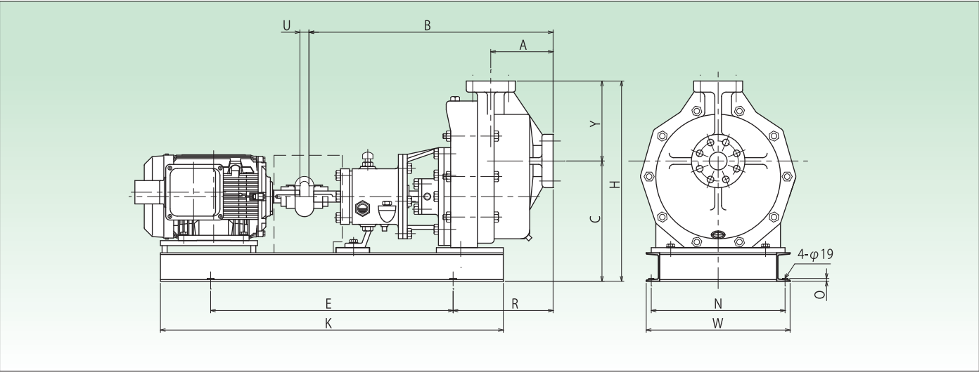
外形寸法図表
