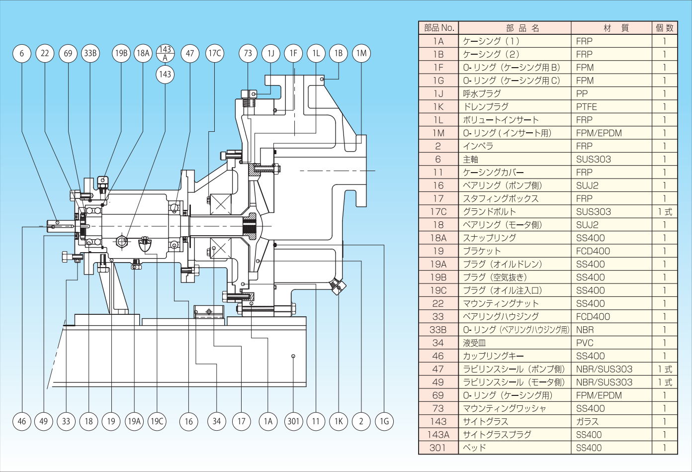
断面構造図
