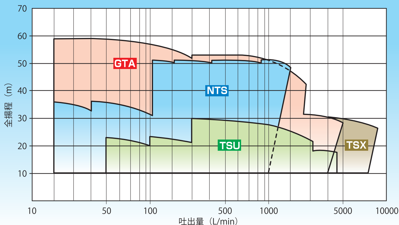
横形ポンプ 50Hz 容量図 〈GTA/TSX/NTS/TSU〉
