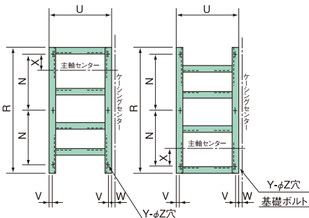
RH2、RL2形基礎図 (A-A視)
