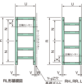
RL形基礎図
