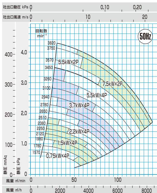
容量図
