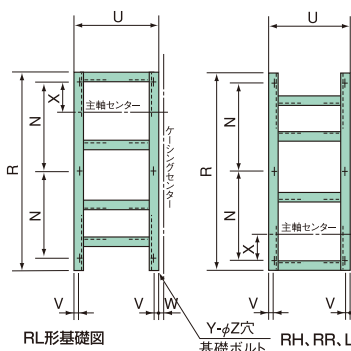
RL形基礎図
