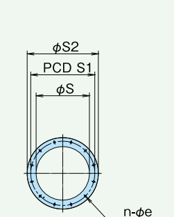
送風機吸込フランジ詳細
