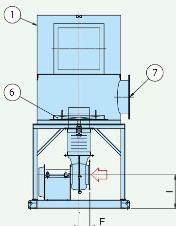
送風機吸込フランジ詳細
