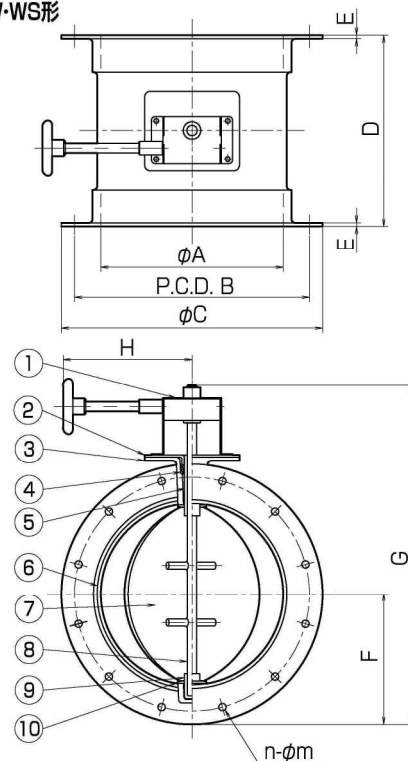
■FDP-100~500-WS形部品表
